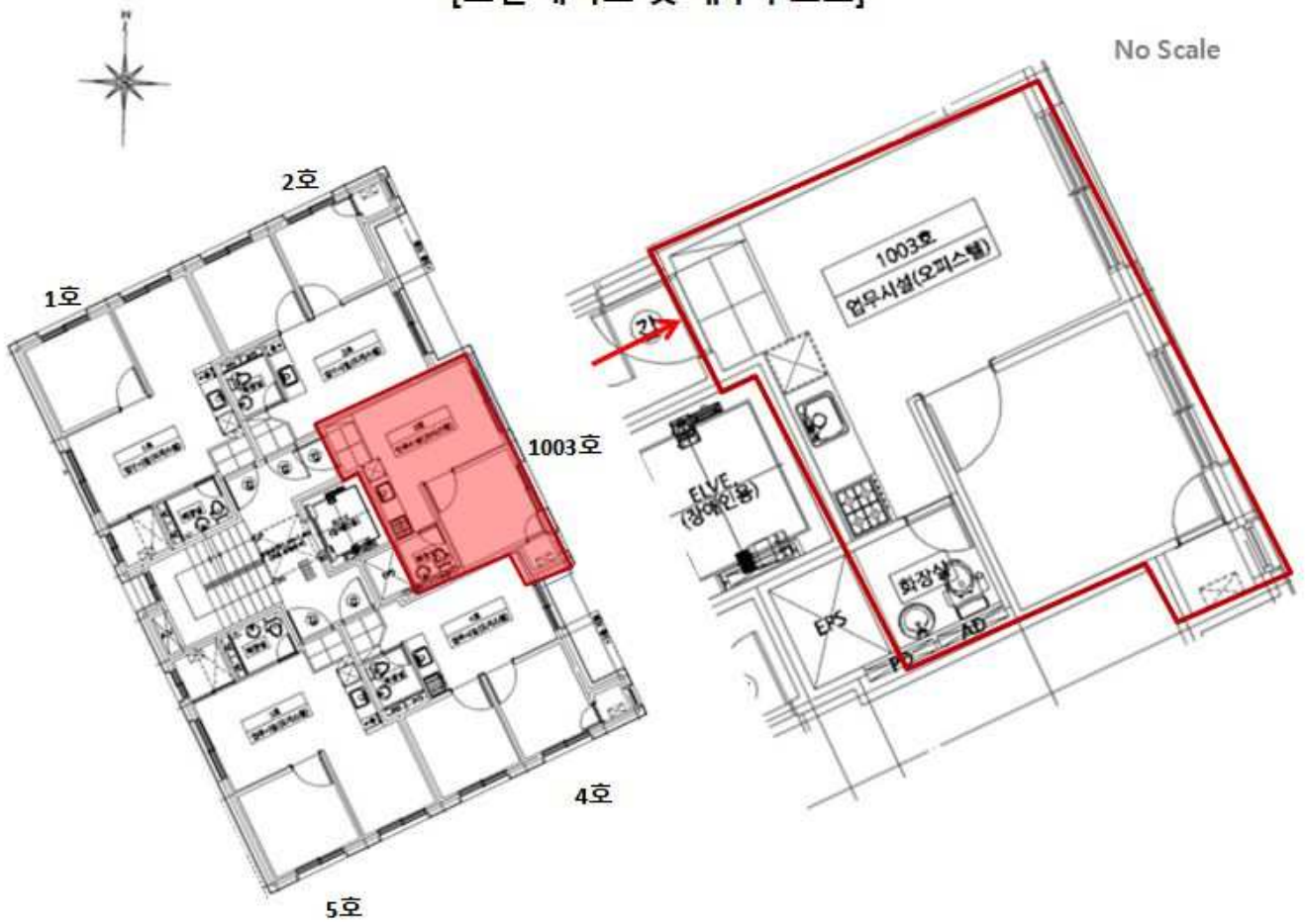
<제10층 호별배치도>
