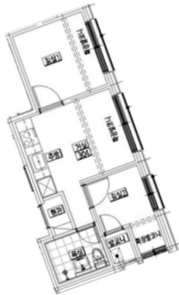
< 호별 배치도 >
