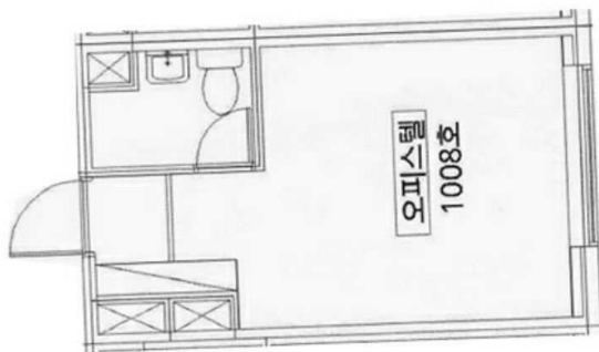
내부구조도(제1008호)
