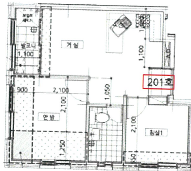
[ 내부구조도 ]
