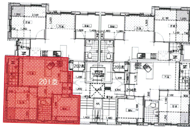
[ 호별배치도 ]
