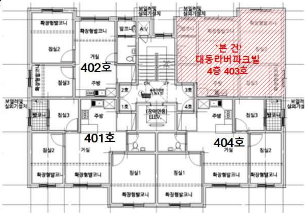
내부구조도(4층 403호)
