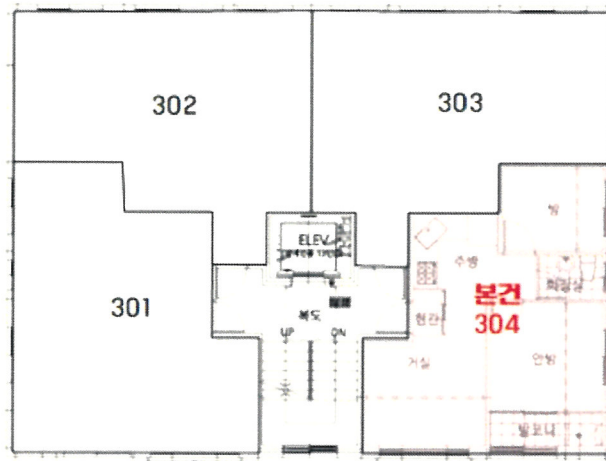
[서울특별시 강서구 화곡동 162-7외 1필지 하나아이파크빌 제3층 호별배치도]
