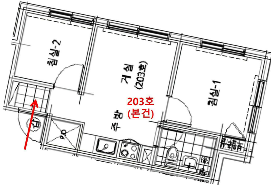
[내부 구조도]
