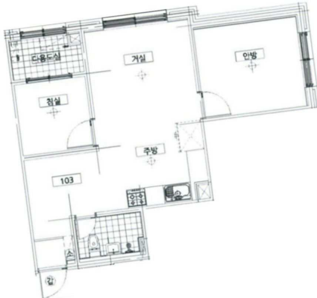
[내부구조도]
