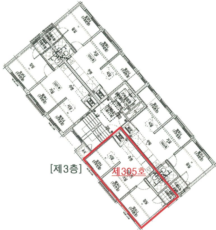
호별배치도
