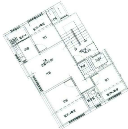
[내부구조도]
