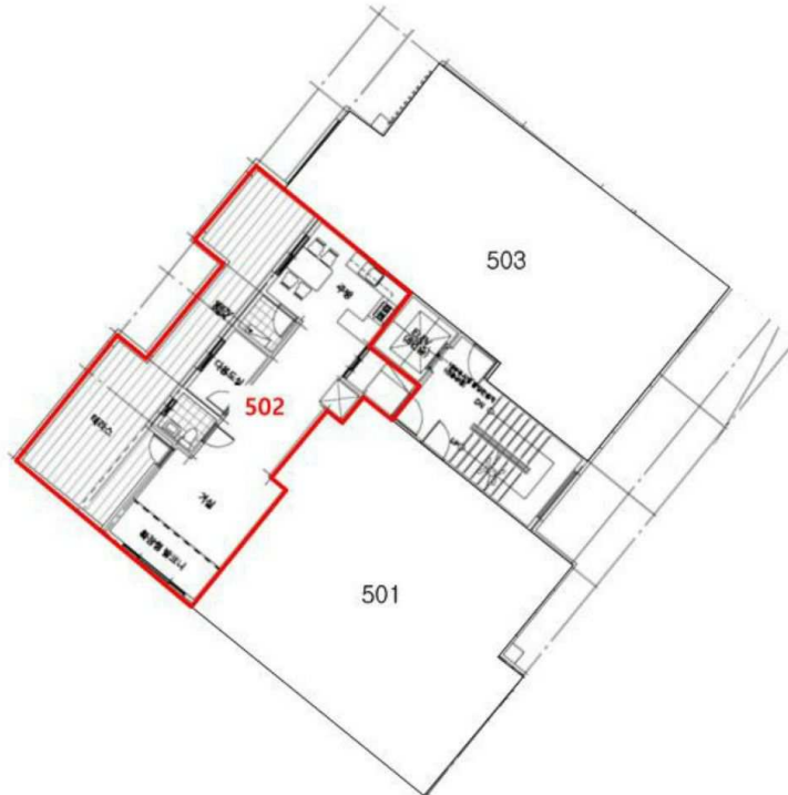
호별배치도
