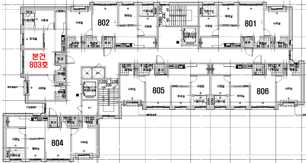
[제8층 층별배치도]
