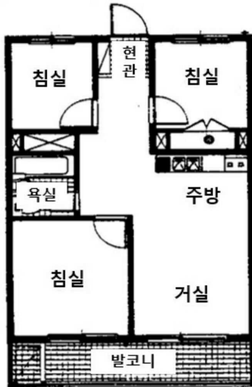
[본건 내부구조도]
