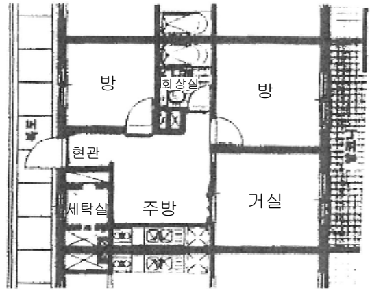
<내부구조도>
