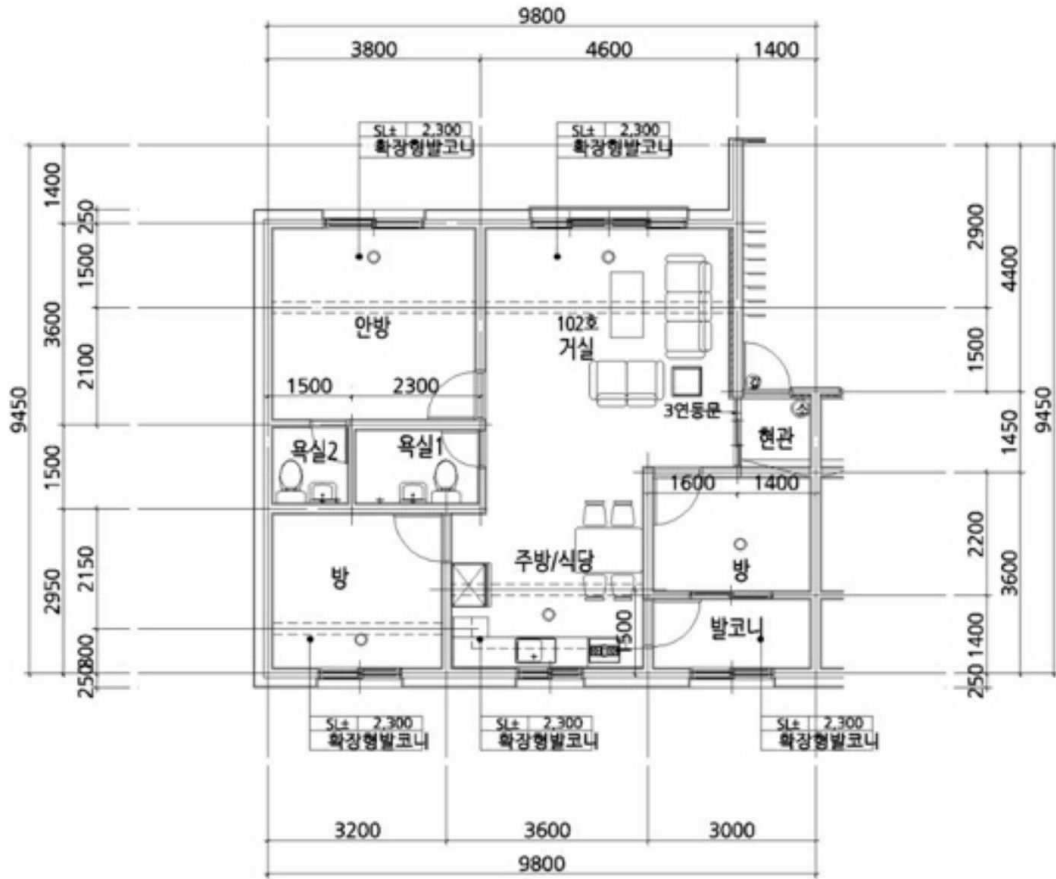
<내부구조도>
