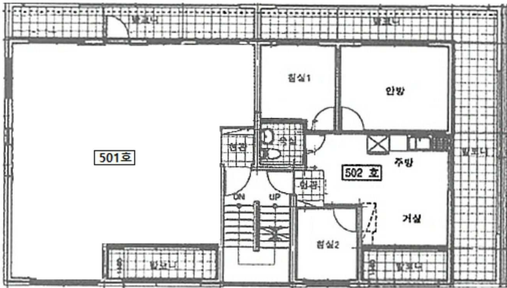
<건축물현황도상 내부구조도>
