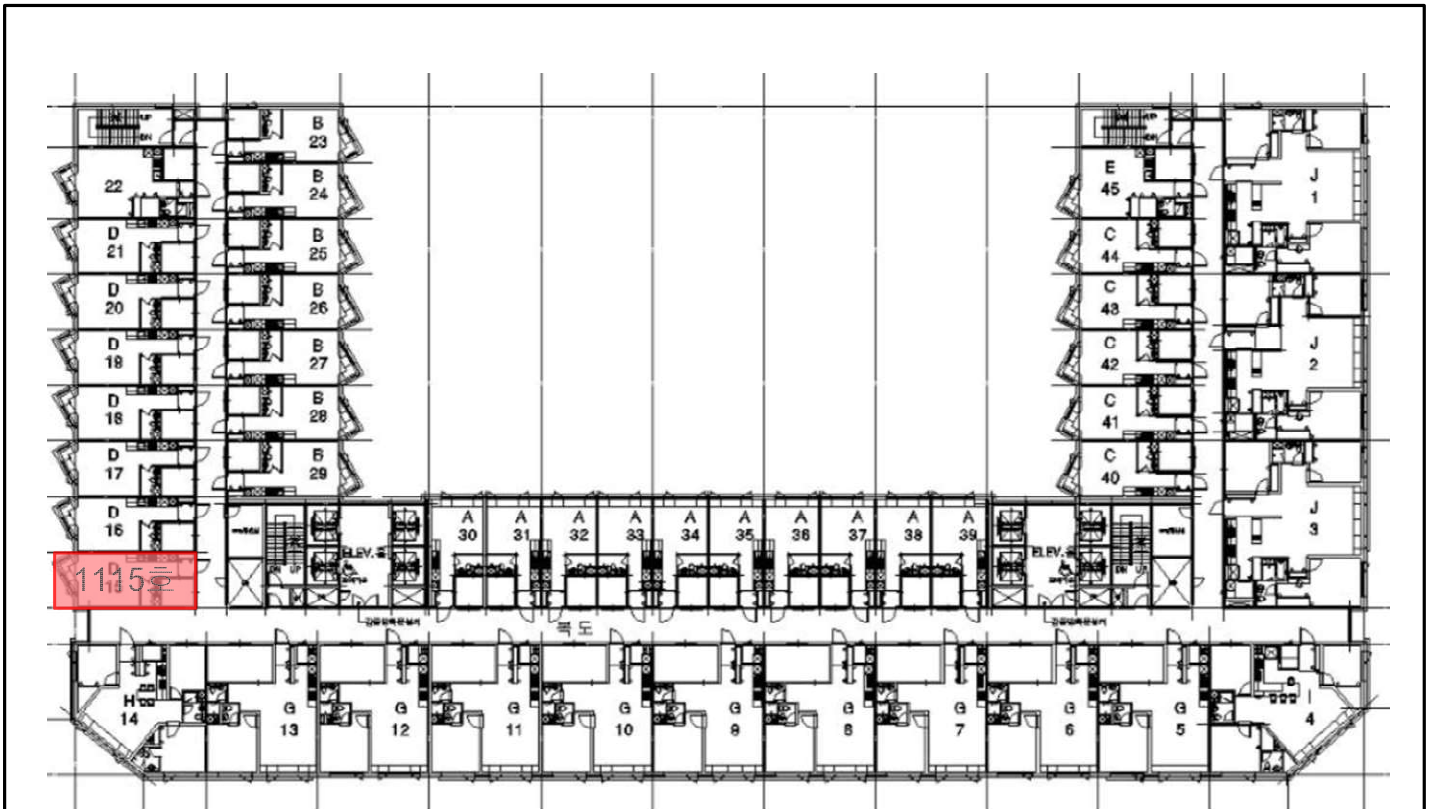
< 우림로데오스위트 제11층 층별 배치도 >
