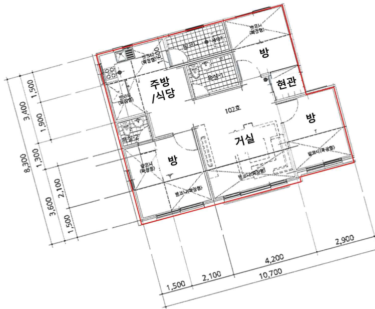
[내부구조도]
