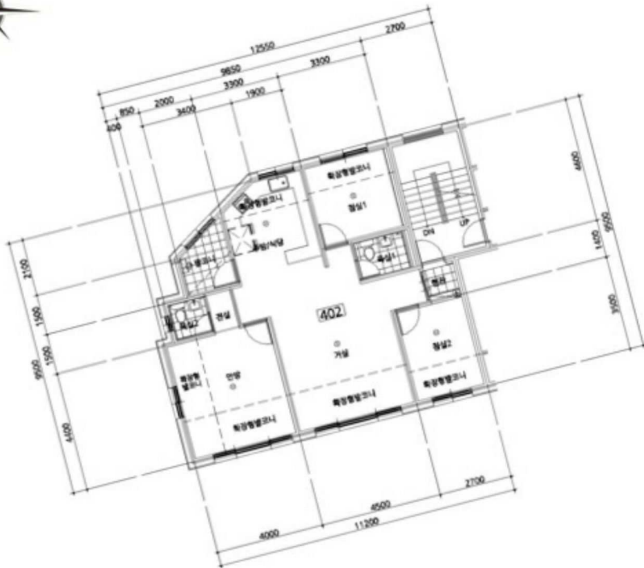
<내부구조도>
