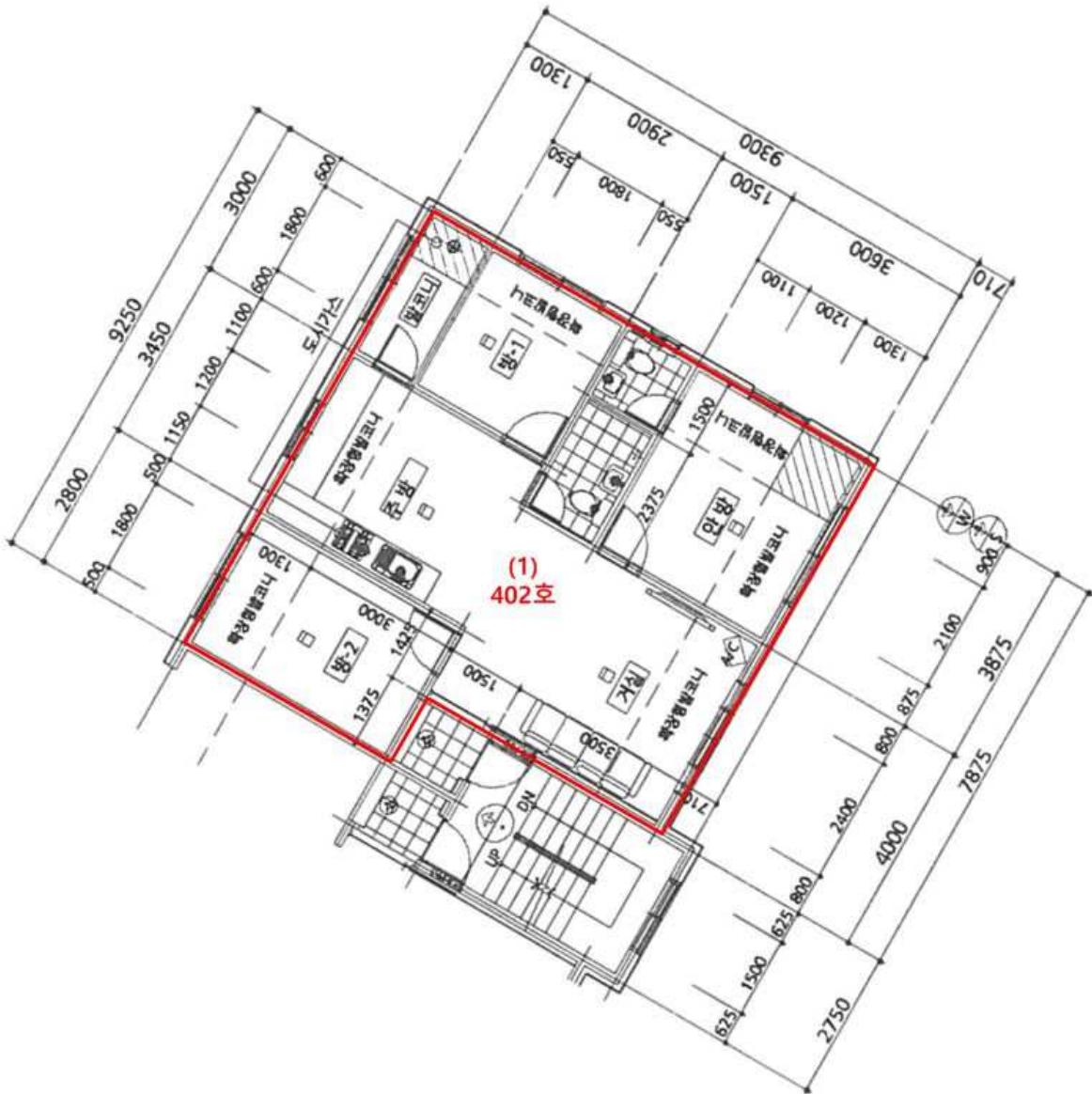
[ 내부구조도 ]
