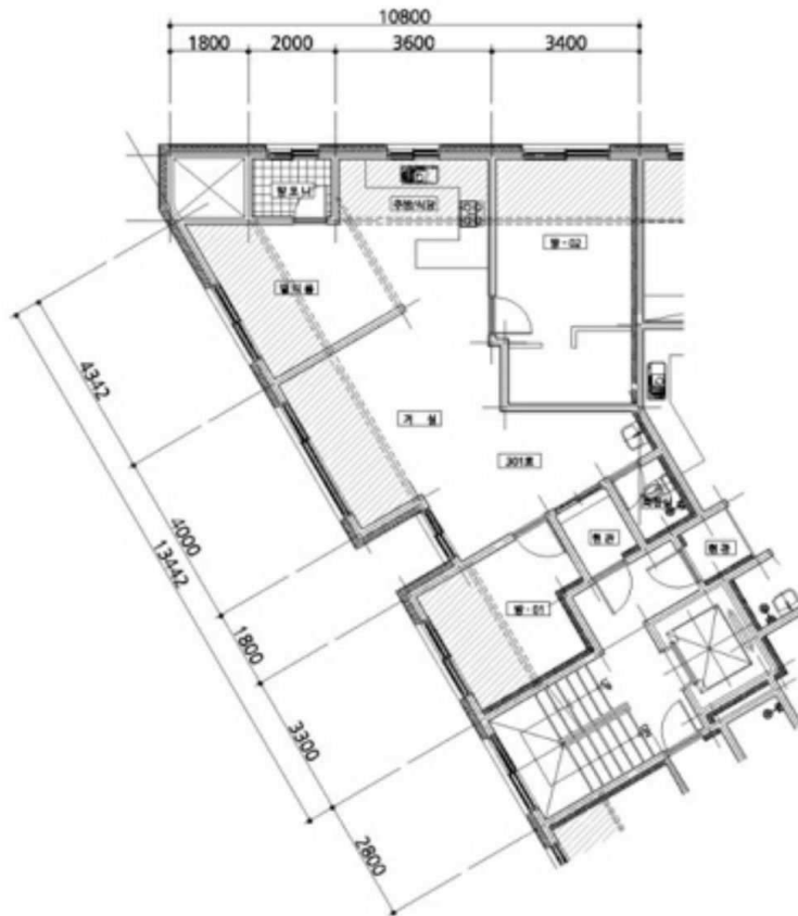
<내부구조도>
