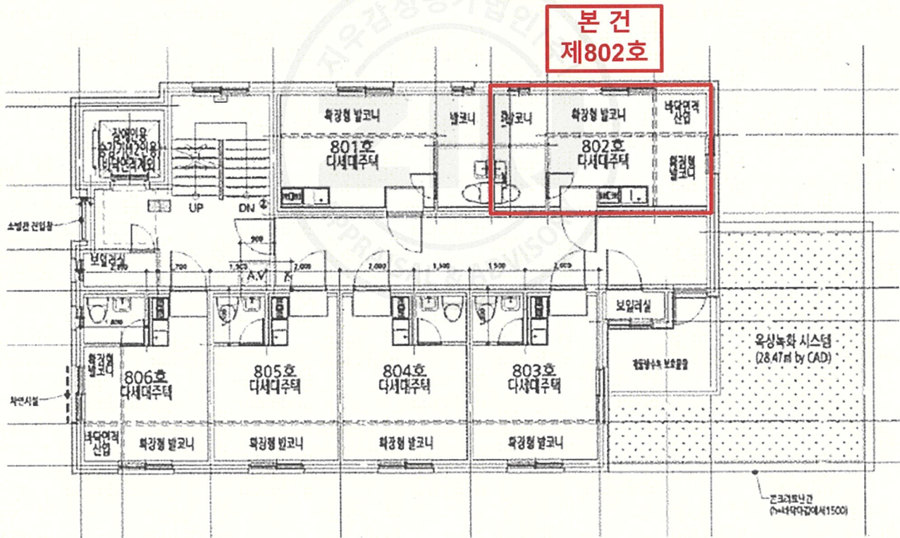
[ 태양오피스텔 제8층 ]
