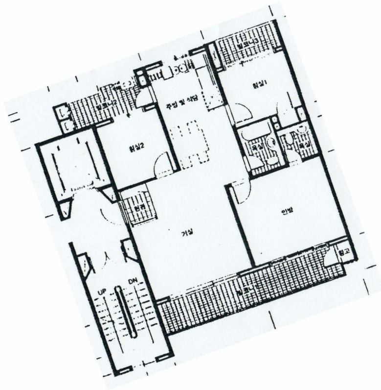
내부구조도
