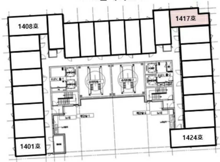
< 내부구조도 >
