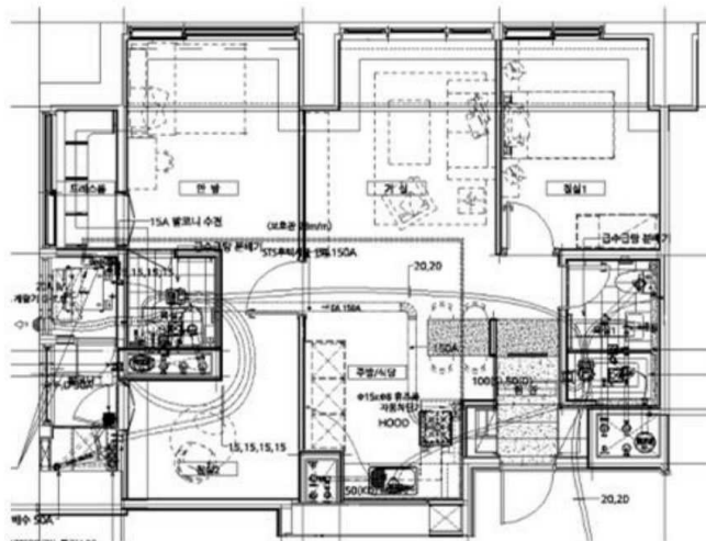
< 건축물현황도상 호별배치도 >
