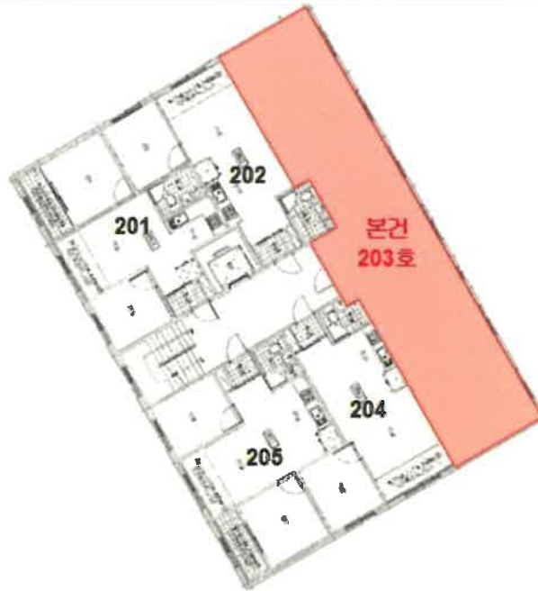
< 씨니빌리지 제2층 호별배치도 >
