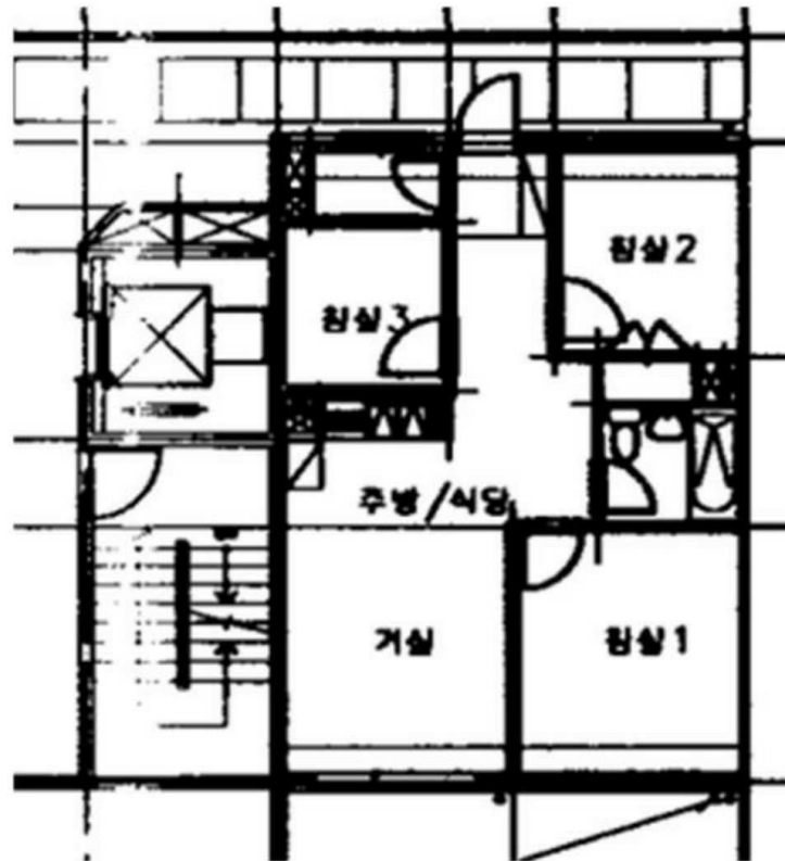
< 건축물현황도상 내부구조도 >
