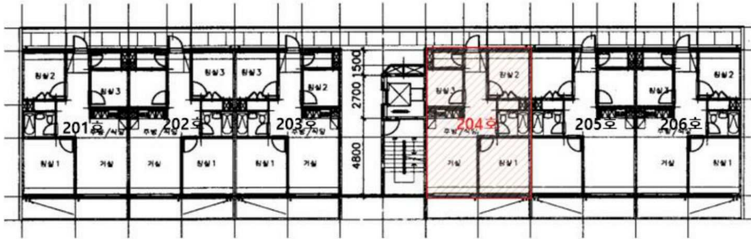
< 건축물현황도상 호별배치도 >
