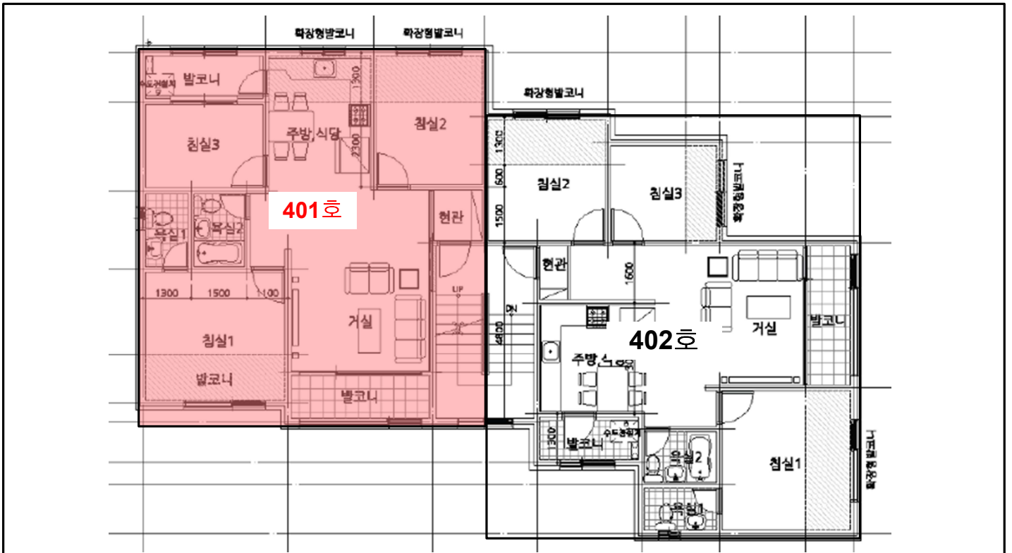
< 상지석동 133-34 제116동 제4층 층별 배치도 >
