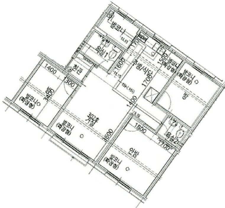
[ 청우하이츠 제106동 제3층 제302호 내부구조도 ]
