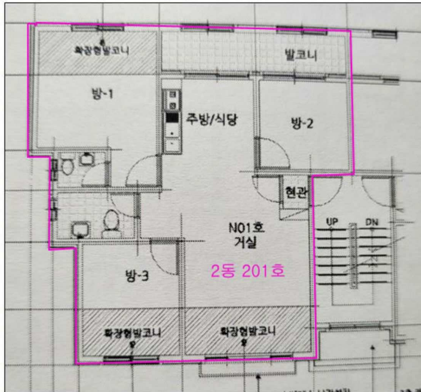
[층별 배치도]
