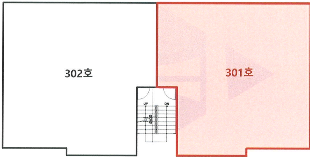
<제3층 호별배치도>
