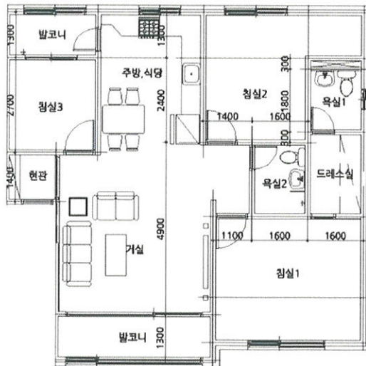
<제3층 제301호 내부구조도>
