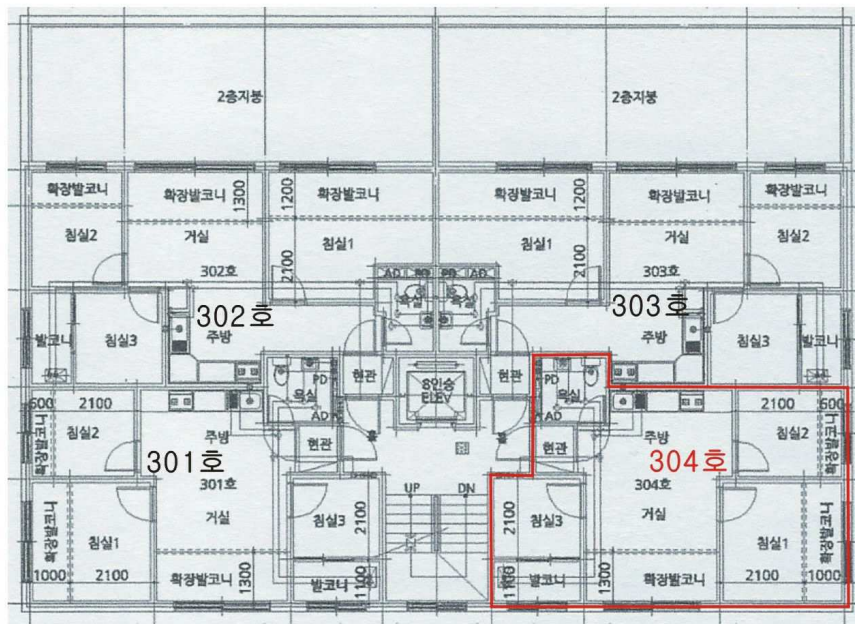
(호별배치도)
