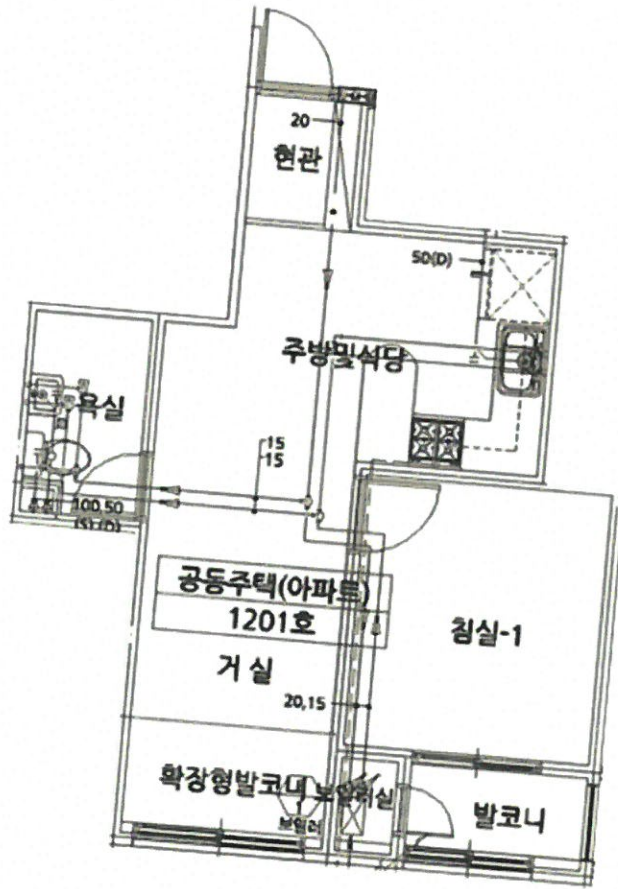
< 내부구조도 >
