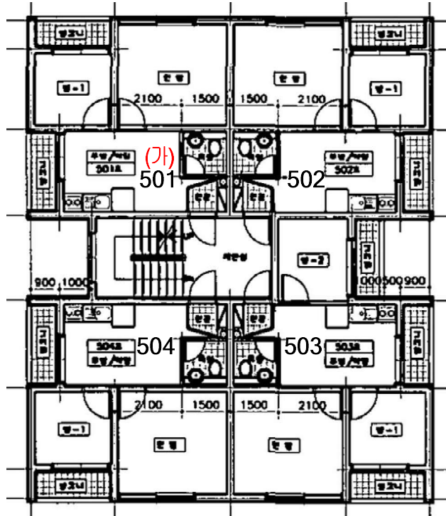
[내부구조도]
