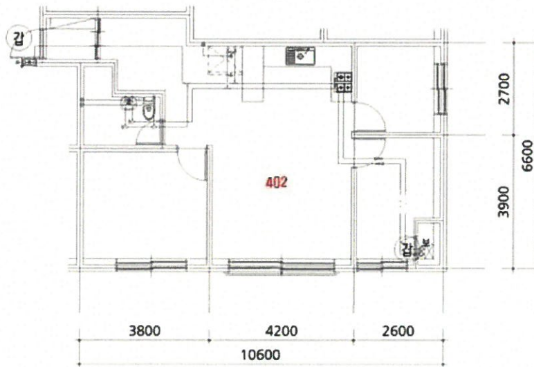
<내부구조도>
