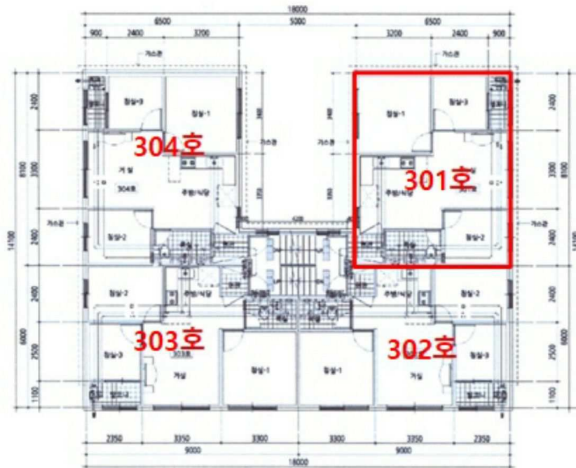
<제3층 평면도 >
