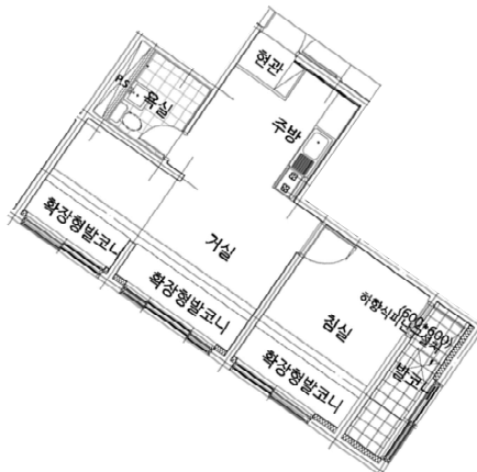
〈내부구조도〉
