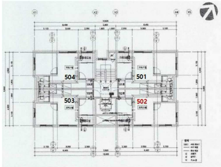
[호별배치도]
