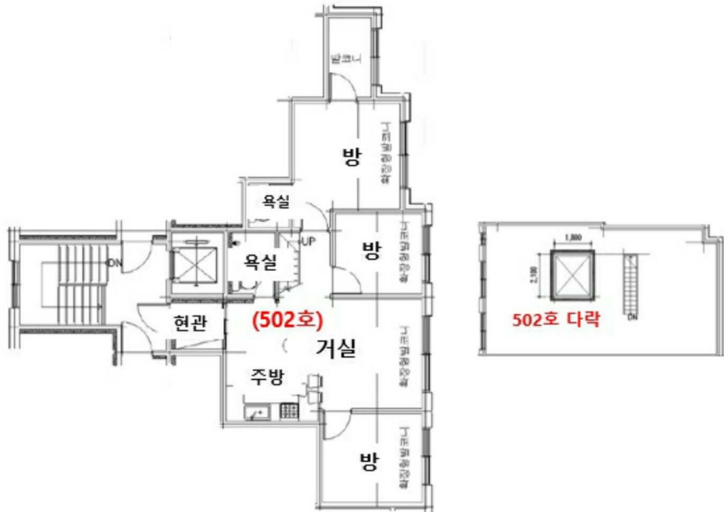
[내부구조도]
