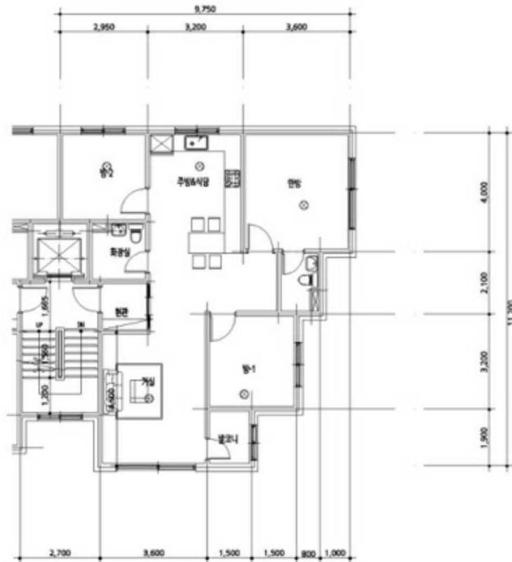
<내부구조도>
