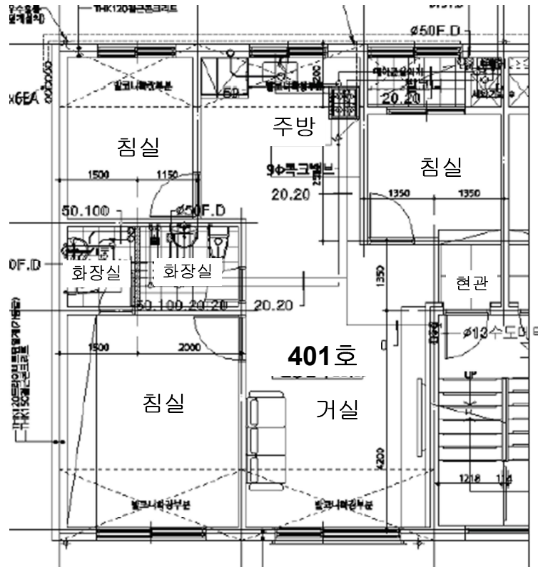
<스페이스 제105동 제4층 제401호 내부 구조도>
