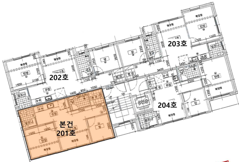
[내부구조도]
