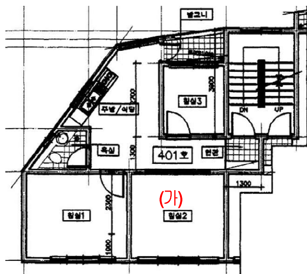
[내부구조도]
