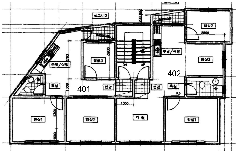
[내부구조도]
