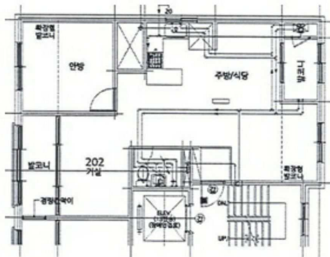
[내부구조도]
