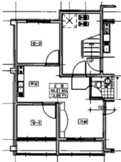
[내부구조도]
