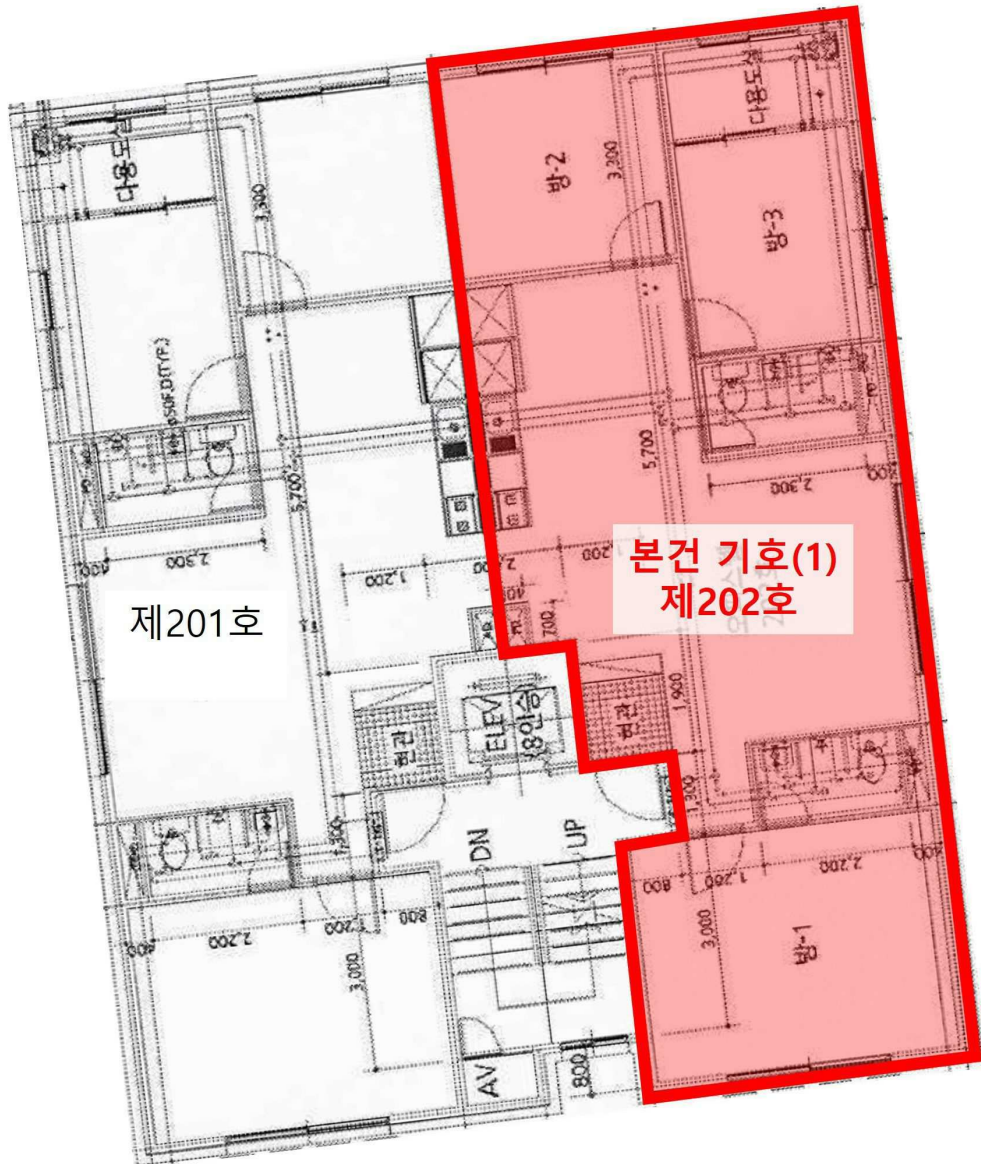
[ 모던하우스 제2층 호별배치도 ]
