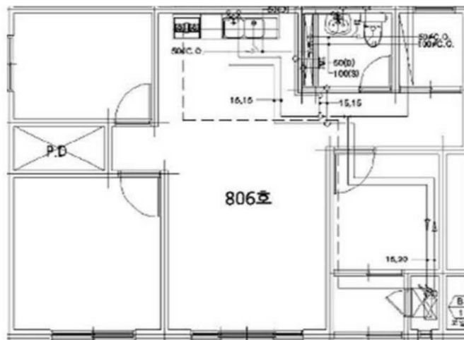
[ 내부구조도 ]
