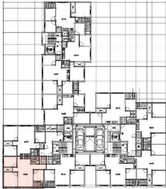
[ 호별배치도 ]
