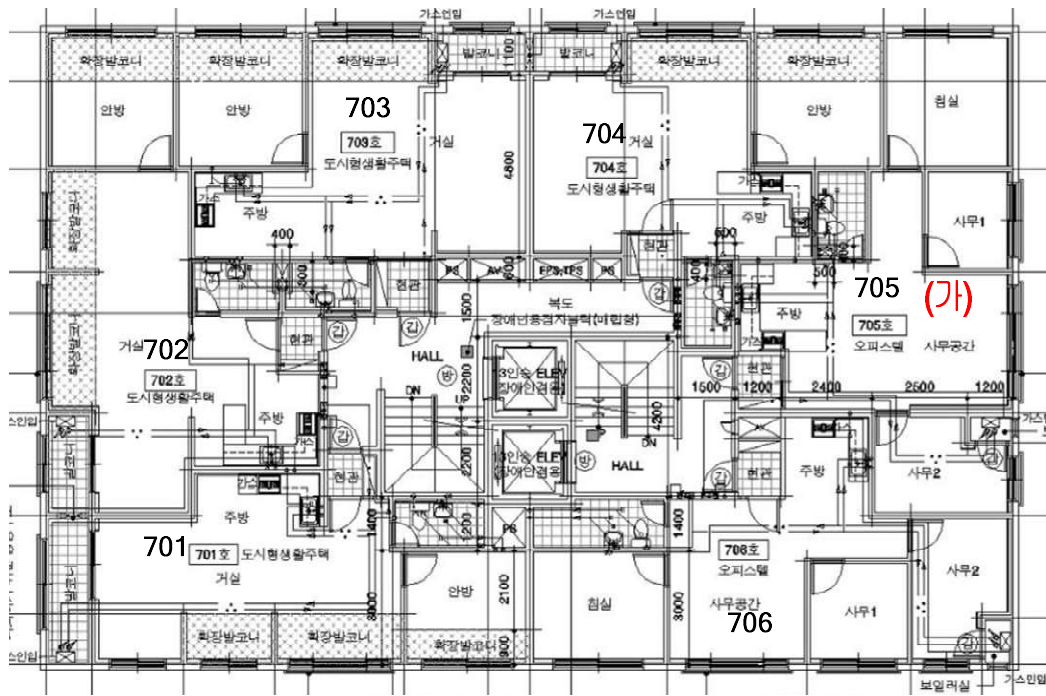
[내부구조도]
