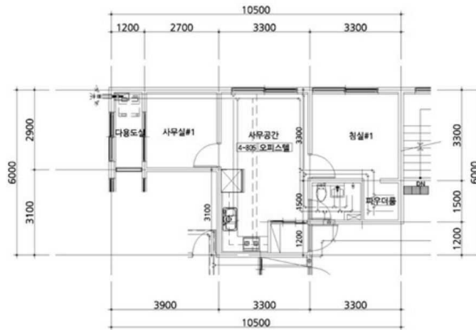
< 4층 405호 내부구조도 >
