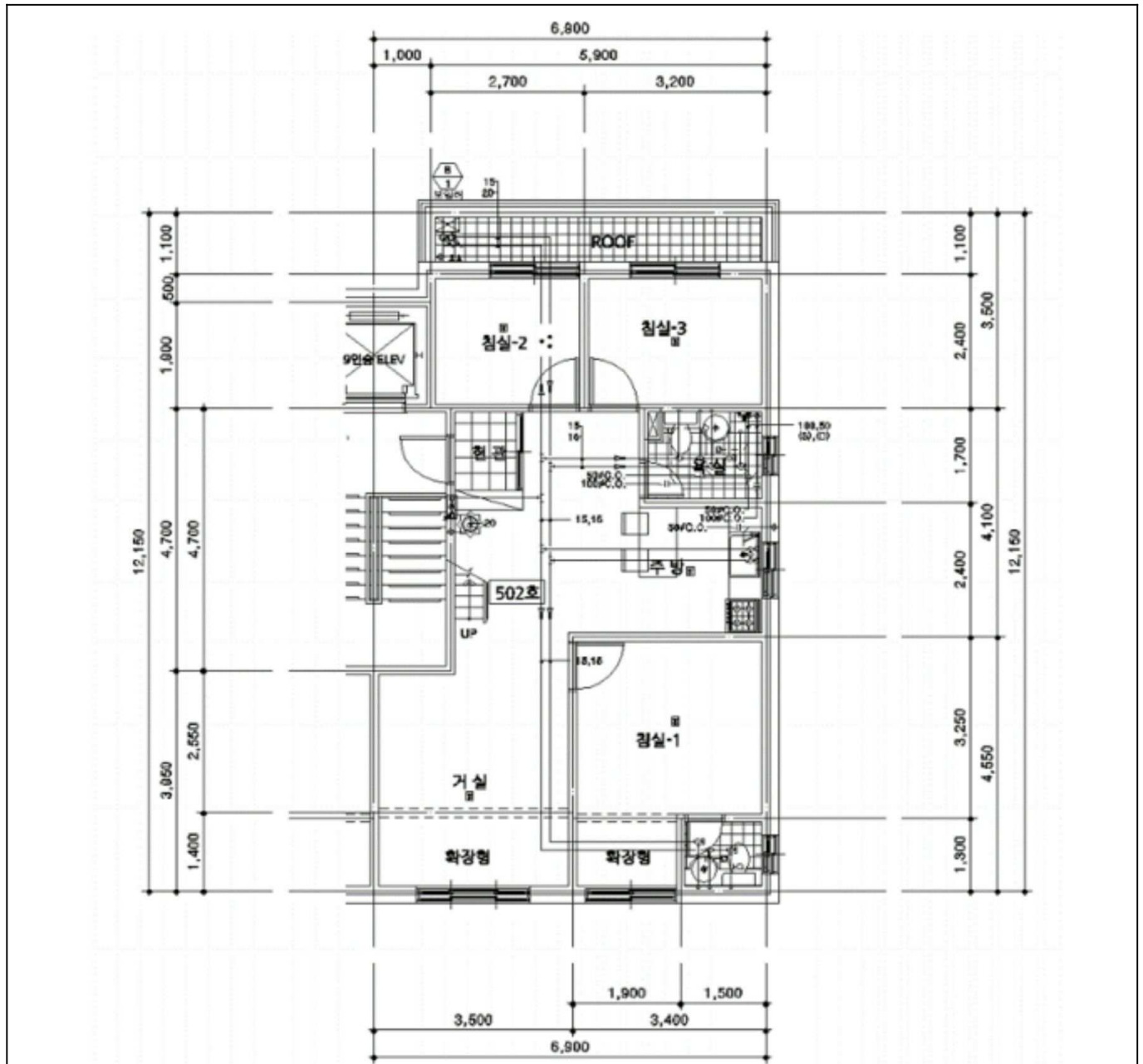
[내부구조도]
